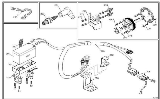
ENCENDIDO Y CONJUNTO ELÉCTRICO
